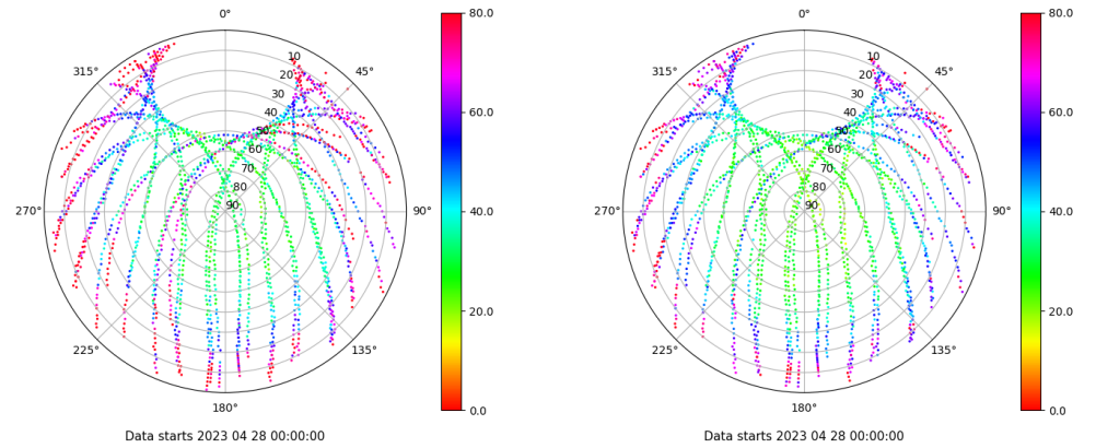
Skyplot for station SEV1. Parameter M1C Data file SEV100ESP_R_2023118.xtr Skyplot for station SEV1. Parameter M2C Data file SEV100ESP_R_2023118.xtr
