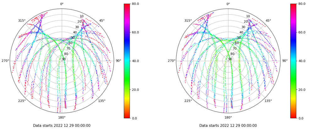
Skyplot for station SEV1. Parameter M1C Data file SEV100ESP_R_2022363.xtr Skyplot for station SEV1. Parameter M2C Data file SEV100ESP_R_2022363.xtr
