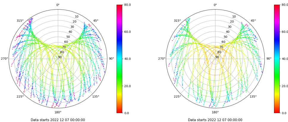
Skyplot for station SEV1. Parameter M1C Data file SEV100ESP_R_2022341.xtr Skyplot for station SEV1. Parameter M2X Data file SEV100ESP_R_2022341.xtr
