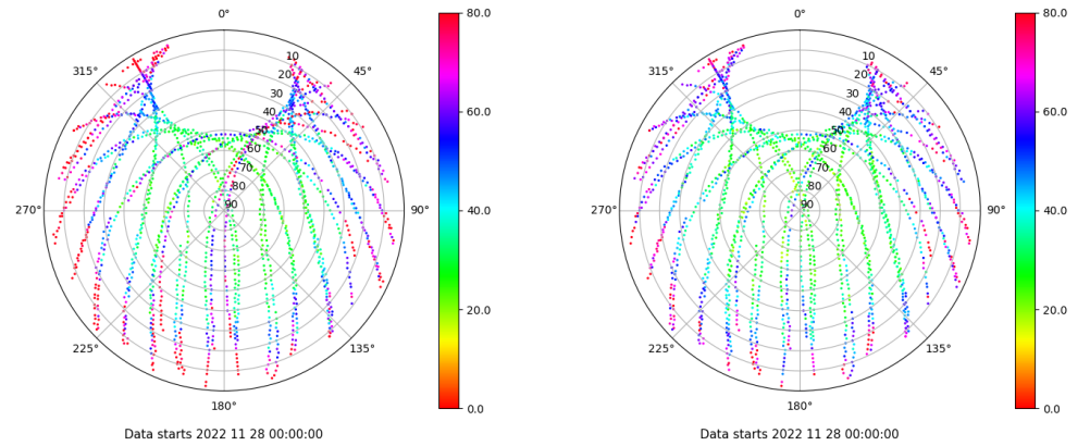
Skyplot for station SEV1. Parameter M1C Data file SEV100ESP_R_2022332.xtr Skyplot for station SEV1. Parameter M2C Data file SEV100ESP_R_2022332.xtr
