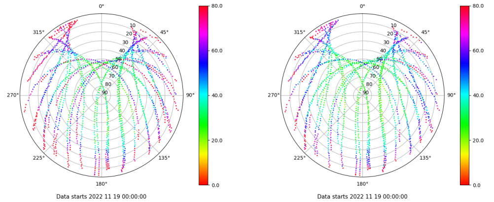
Skyplot for station SEV1. Parameter M1C Data file SEV100ESP_R_2022323.xtr Skyplot for station SEV1. Parameter M2C Data file SEV100ESP_R_2022323.xtr
