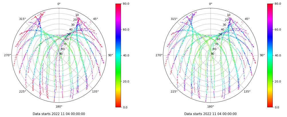
Skyplot for station SEV1. Parameter M1C Data file SEV100ESP_R_2022308.xtr Skyplot for station SEV1. Parameter M2C Data file SEV100ESP_R_2022308.xtr
