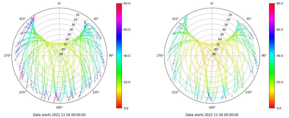
Skyplot for station SEV1. Parameter M1C Data file SEV100ESP_R_2022308.xtr Skyplot for station SEV1. Parameter M2X Data file SEV100ESP_R_2022308.xtr
