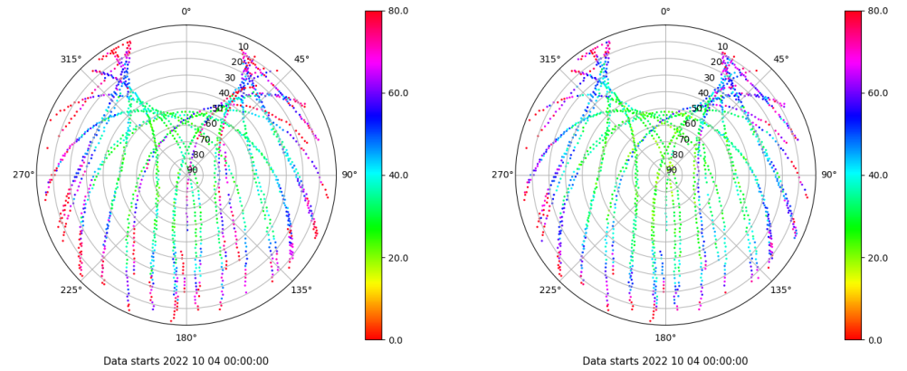
Skyplot for station SEV1. Parameter M1C Data file SEV100ESP_R_2022277.xtr Skyplot for station SEV1. Parameter M2C Data file SEV100ESP_R_2022277.xtr
