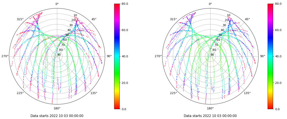
Skyplot for station SEV1. Parameter M1C Data file SEV100ESP_R_2022276.xtr Skyplot for station SEV1. Parameter M2C Data file SEV100ESP_R_2022276.xtr
