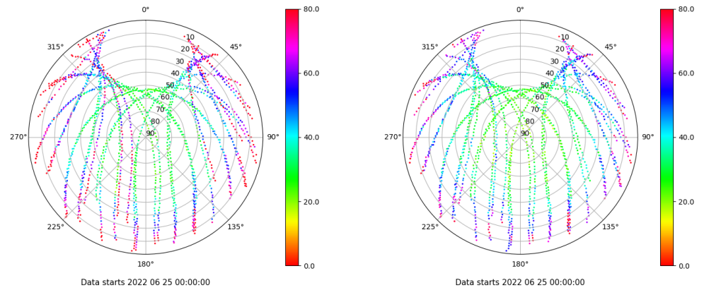
Skyplot for station SEV1. Parameter M1C Data file SEV100ESP_R_2022176.xtr Skyplot for station SEV1. Parameter M2C Data file SEV100ESP_R_2022176.xtr
