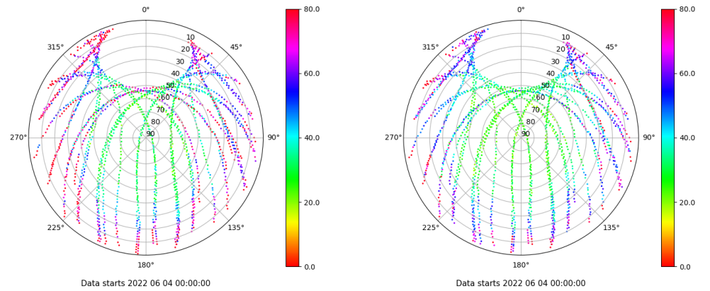
Skyplot for station SEV1. Parameter M1C Data file SEV100ESP_R_2022155.xtr Skyplot for station SEV1. Parameter M2C Data file SEV100ESP_R_2022155.xtr
