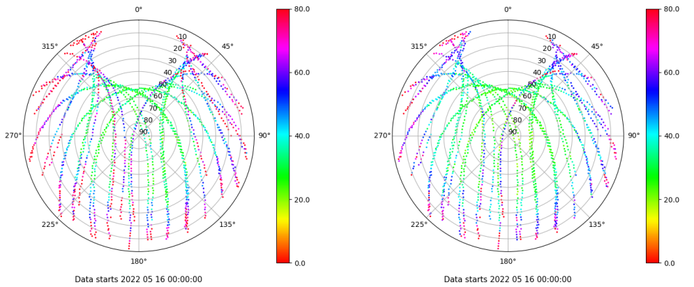
Skyplot for station SEV1. Parameter M1C Data file SEV100ESP_R_2022136.xtr Skyplot for station SEV1. Parameter M2C Data file SEV100ESP_R_2022136.xtr
