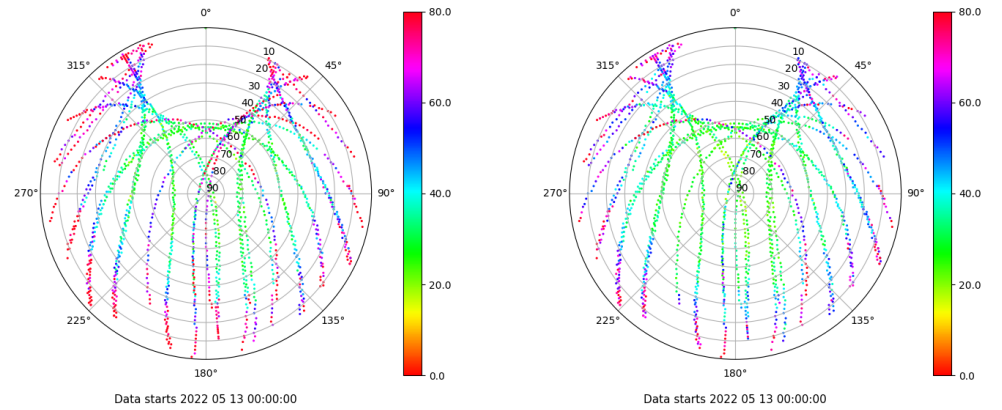
Skyplot for station SEV1. Parameter M1C Data file SEV100ESP_R_2022133.xtr Skyplot for station SEV1. Parameter M2C Data file SEV100ESP_R_2022133.xtr
