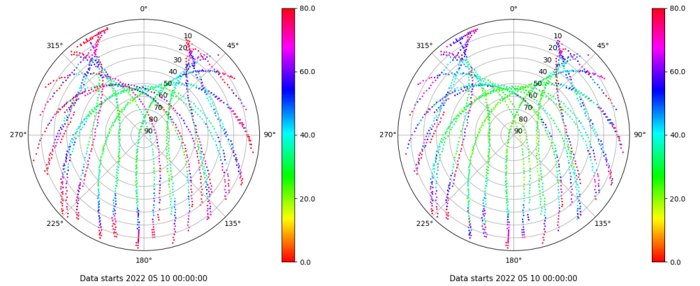
Skyplot for station SEV1. Parameter M1C Data file SEV100ESP_R_2022130.xtr Skyplot for station SEV1. Parameter M2C Data file SEV100ESP_R_2022130.xtr
