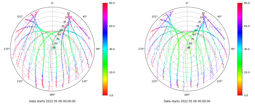
Skyplot for station SEV1. Parameter M1C Data file SEV100ESP_R_2022126.xtr Skyplot for station SEV1. Parameter M2C Data file SEV100ESP_R_2022126.xtr
