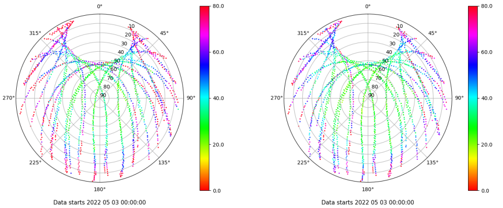
Skyplot for station SEV1. Parameter M1C Data file SEV100ESP_R_2022123.xtr Skyplot for station SEV1. Parameter M2C Data file SEV100ESP_R_2022123.xtr
