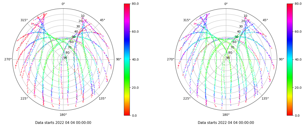
Skyplot for station SEV1. Parameter M1C Data file SEV100ESP_R_2022094.xtr Skyplot for station SEV1. Parameter M2C Data file SEV100ESP_R_2022094.xtr
