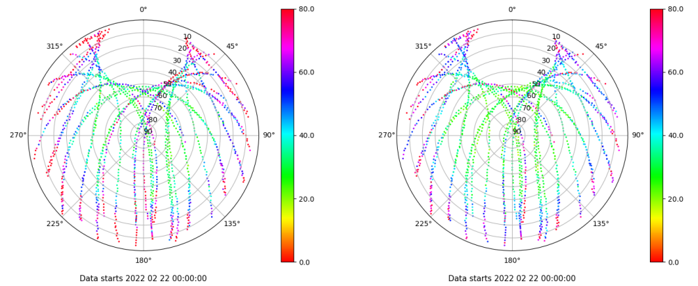
Skyplot for station SEV1. Parameter M1C Data file SEV100ESP_R_2022053.xtr Skyplot for station SEV1. Parameter M2C Data file SEV100ESP_R_2022053.xtr
