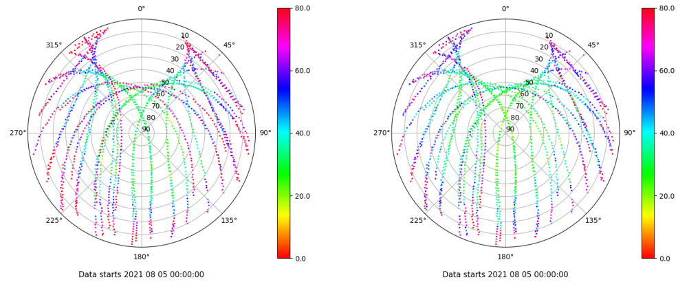
Skyplot for station SEV1. Parameter M1C Data file SEV100ESP_R_2021217.xtr Skyplot for station SEV1. Parameter M2C Data file SEV100ESP_R_2021217.xtr
