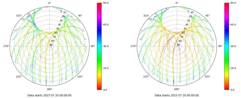
Skyplot for station SALA. Parameter M1C Data file SALA00ESP_R_2023201.xtr Skyplot for station SALA. Parameter M2P Data file SALA00ESP_R_2023201.xtr
