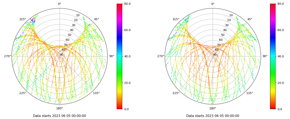
Skyplot for station SALA. Parameter M1C Data file SALA00ESP_R_2023156.xtr Skyplot for station SALA. Parameter M2S Data file SALA00ESP_R_2023156.xtr
