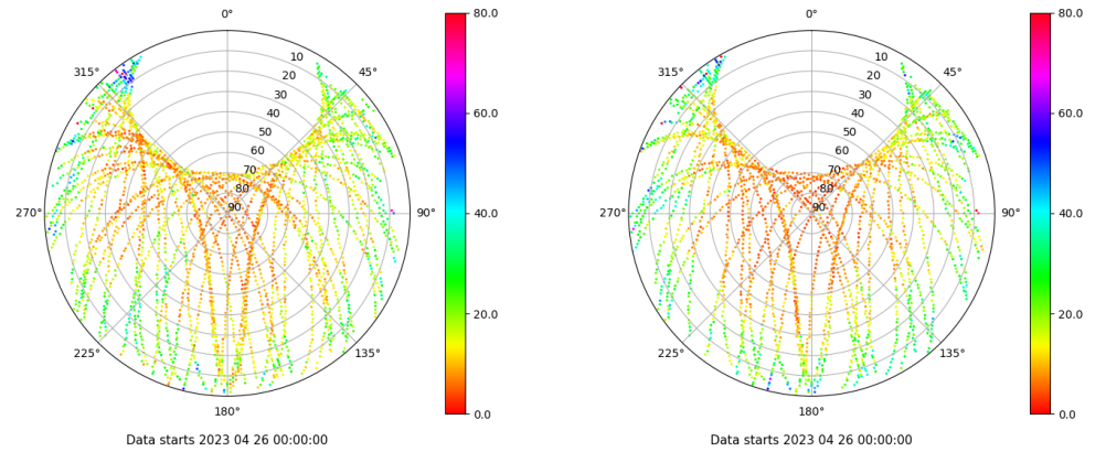
Skyplot for station SALA. Parameter M1C Data file SALA00ESP_R_2023116.xtr Skyplot for station SALA. Parameter M2S Data file SALA00ESP_R_2023116.xtr
