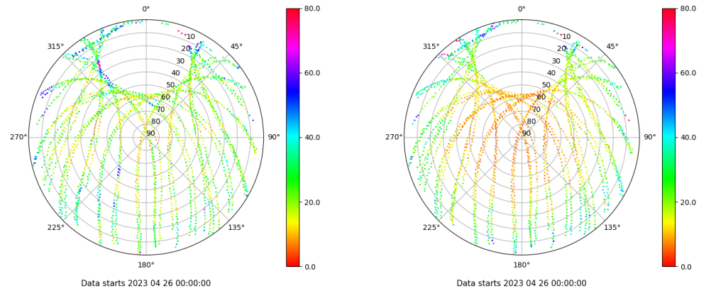
Skyplot for station SALA. Parameter M1C Data file SALA00ESP_R_2023116.xtr Skyplot for station SALA. Parameter M2P Data file SALA00ESP_R_2023116.xtr
