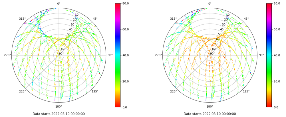
Skyplot for station SALA. Parameter M1C Data file SALA00ESP_R_2022069.xtr Skyplot for station SALA. Parameter M2P Data file SALA00ESP_R_2022069.xtr
