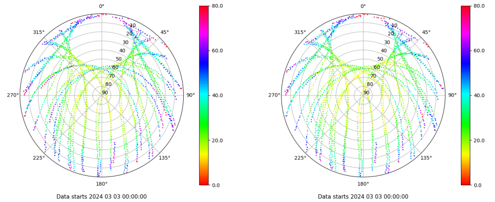
Skyplot for station RODI. Parameter M1C Data file RODI00ESP_R_2024063.xtr Skyplot for station RODI. Parameter M2C Data file RODI00ESP_R_2024063.xtr
