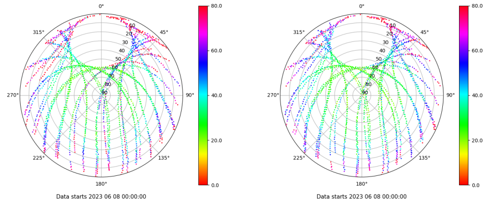
Skyplot for station RODI. Parameter M1C Data file RODI00ESP_R_2023159.xtr Skyplot for station RODI. Parameter M2C Data file RODI00ESP_R_2023159.xtr
