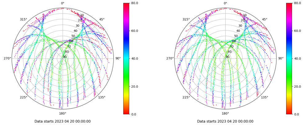
Skyplot for station RODI. Parameter M1C Data file RODI00ESP_R_2023110.xtr Skyplot for station RODI. Parameter M2C Data file RODI00ESP_R_2023110.xtr
