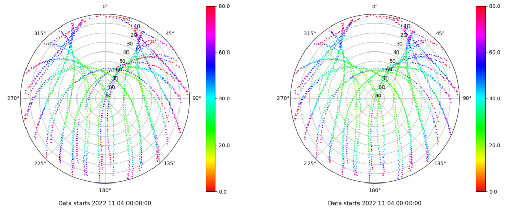
Skyplot for station RODI. Parameter M1C Data file RODI00ESP_R_2022308.xtr Skyplot for station RODI. Parameter M2C Data file RODI00ESP_R_2022308.xtr
