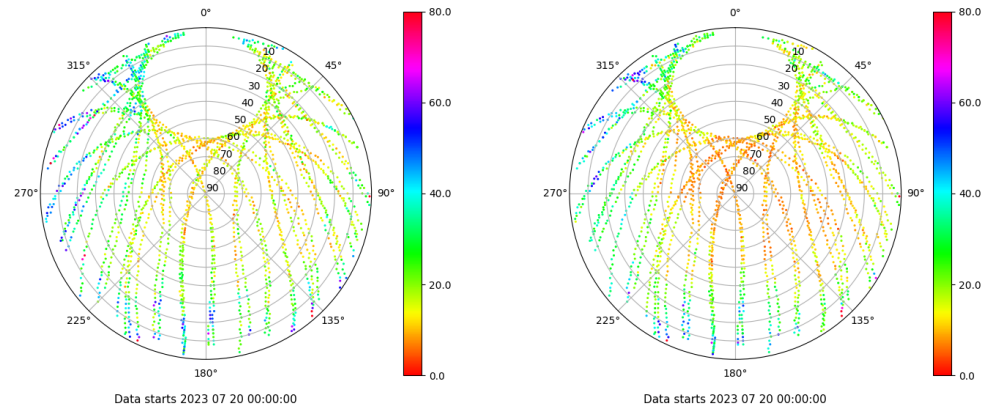
Skyplot for station RIO1. Parameter M1C Data file RIO100ESP_R_2023201.xtr Skyplot for station RIO1. Parameter M2P Data file RIO100ESP_R_2023201.xtr
