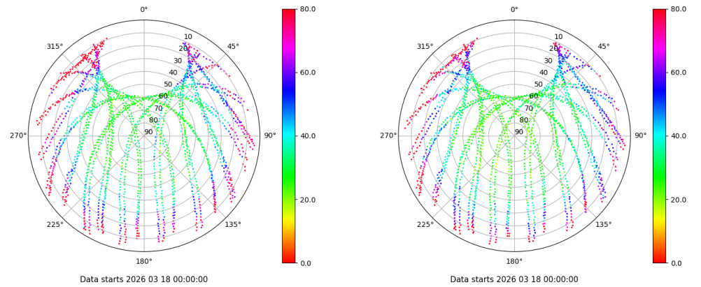
Skyplot for station PUIG. Parameter M1C Data file PUIG00ESP_R_2026077.xtr Skyplot for station PUIG. Parameter M2C Data file PUIG00ESP_R_2026077.xtr
