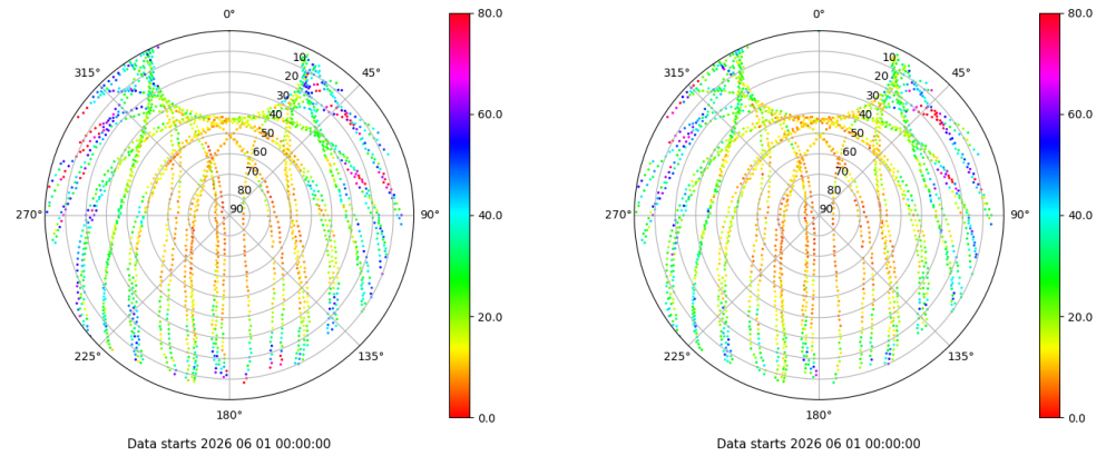
Skyplot for station LPAL. Parameter M1C Data file LPAL00ESP_R_2026152.xtr Skyplot for station LPAL. Parameter M2C Data file LPAL00ESP_R_2026152.xtr
