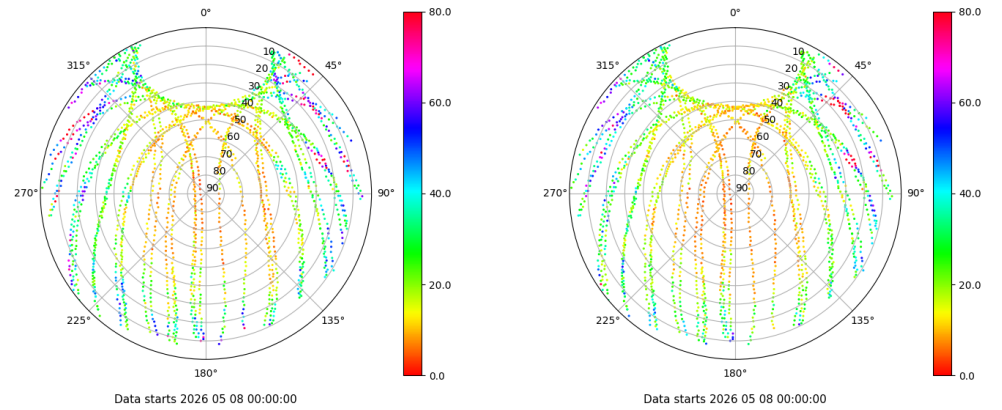
Skyplot for station LPAL. Parameter M1C Data file LPAL00ESP_R_2026128.xtr Skyplot for station LPAL. Parameter M2C Data file LPAL00ESP_R_2026128.xtr
