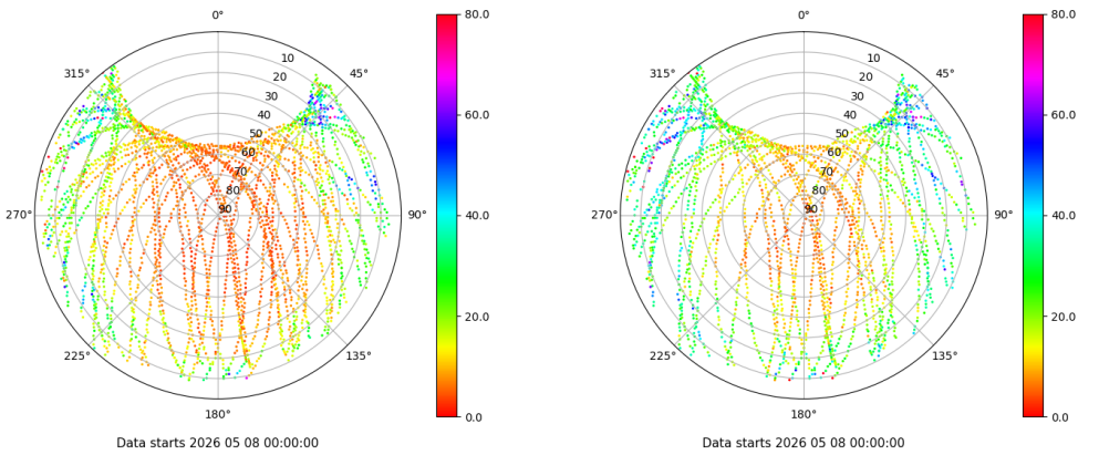
Skyplot for station LPAL. Parameter M1C Data file LPAL00ESP_R_2026128.xtr Skyplot for station LPAL. Parameter M2S Data file LPAL00ESP_R_2026128.xtr
