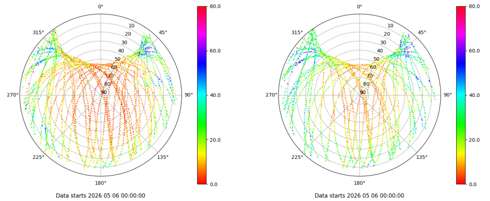
Skyplot for station LPAL. Parameter M1C Data file LPAL00ESP_R_2026126.xtr Skyplot for station LPAL. Parameter M2S Data file LPAL00ESP_R_2026126.xtr
