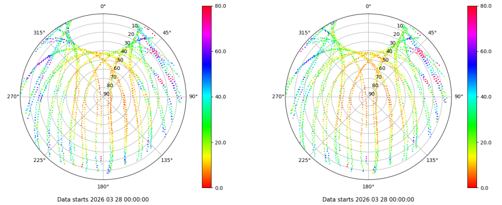
Skyplot for station LPAL. Parameter M1C Data file LPAL00ESP_R_2026087.xtr Skyplot for station LPAL. Parameter M2C Data file LPAL00ESP_R_2026087.xtr
