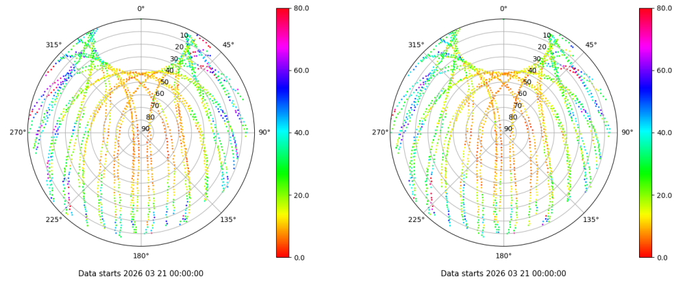
Skyplot for station LPAL. Parameter M1C Data file LPAL00ESP_R_2026080.xtr Skyplot for station LPAL. Parameter M2C Data file LPAL00ESP_R_2026080.xtr
