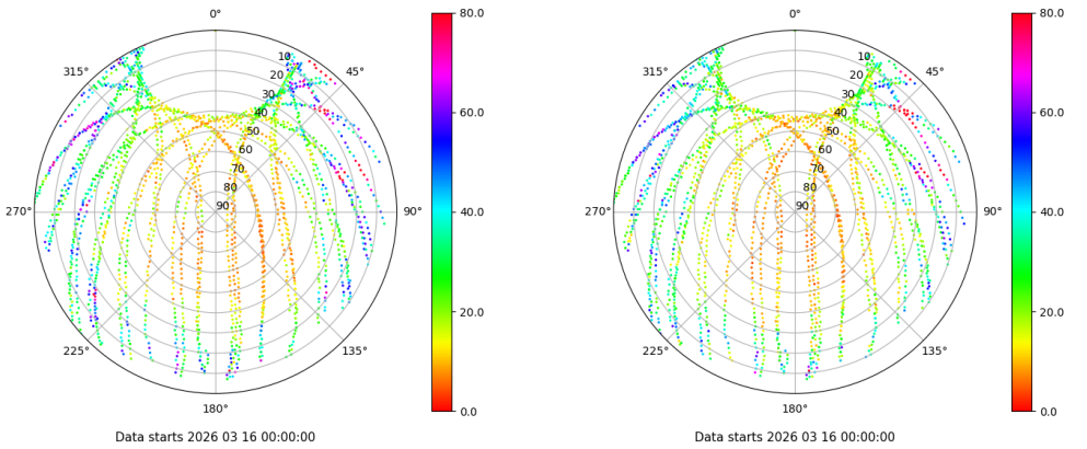
Skyplot for station LPAL. Parameter M1C Data file LPAL00ESP_R_2026075.xtr Skyplot for station LPAL. Parameter M2C Data file LPAL00ESP_R_2026075.xtr
