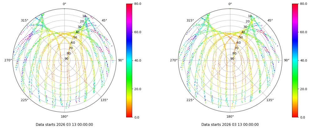
Skyplot for station LPAL. Parameter M1C Data file LPAL00ESP_R_2026072.xtr Skyplot for station LPAL. Parameter M2C Data file LPAL00ESP_R_2026072.xtr
