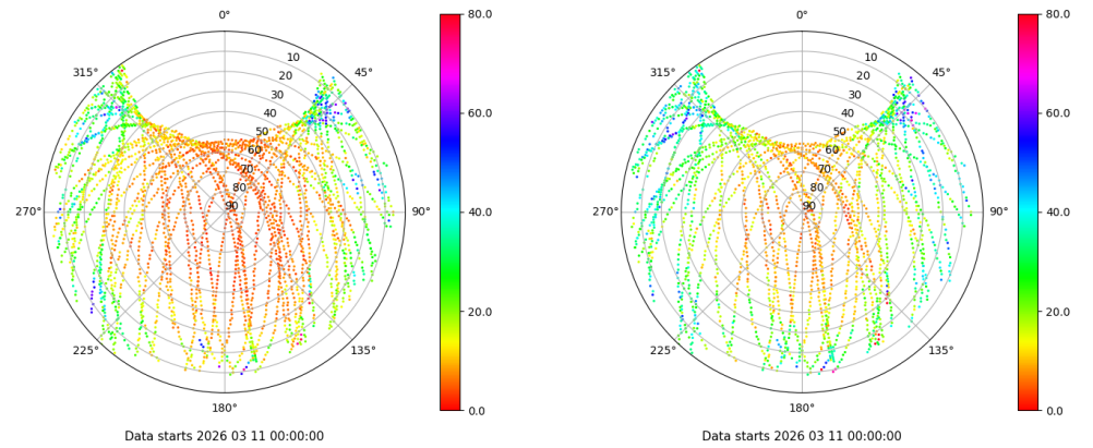
Skyplot for station LPAL. Parameter M1C Data file LPAL00ESP_R_2026070.xtr Skyplot for station LPAL. Parameter M2S Data file LPAL00ESP_R_2026070.xtr
