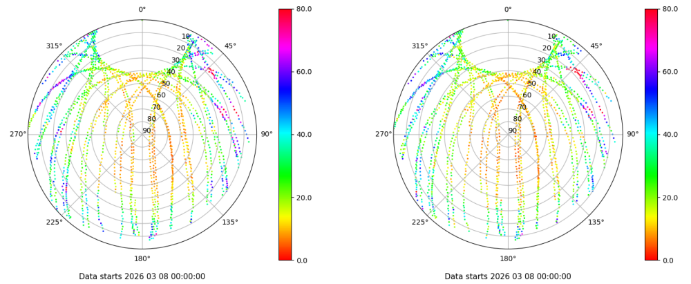
Skyplot for station LPAL. Parameter M1C Data file LPAL00ESP_R_2026067.xtr Skyplot for station LPAL. Parameter M2C Data file LPAL00ESP_R_2026067.xtr
