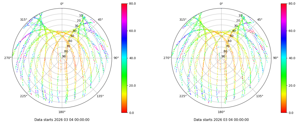
Skyplot for station LPAL. Parameter M1C Data file LPAL00ESP_R_2026063.xtr Skyplot for station LPAL. Parameter M2C Data file LPAL00ESP_R_2026063.xtr
