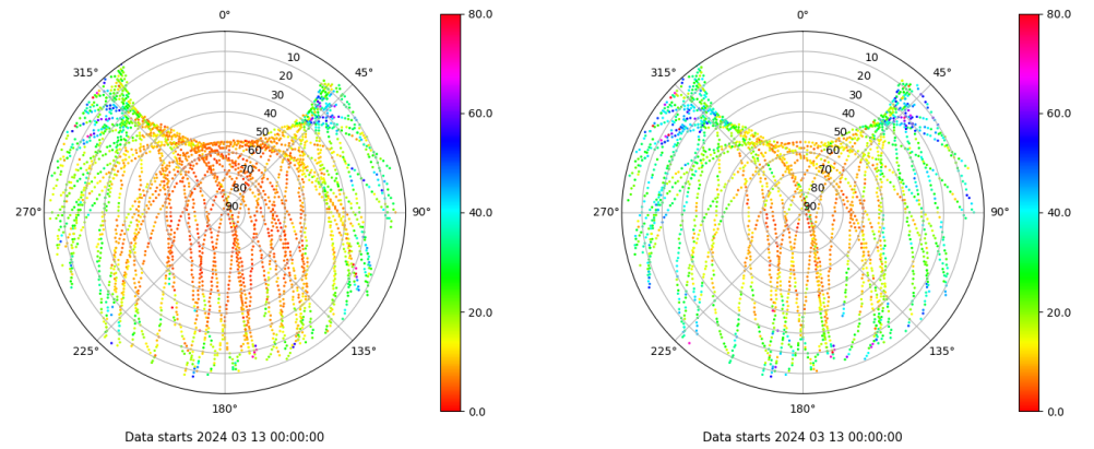
Skyplot for station LPAL. Parameter M1C Data file LPAL00ESP_R_2024073.xtr Skyplot for station LPAL. Parameter M2S Data file LPAL00ESP_R_2024073.xtr
