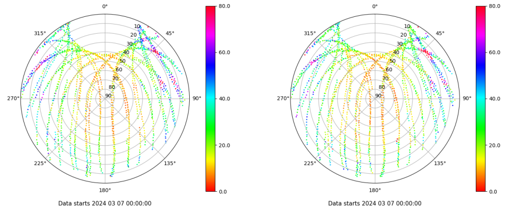
Skyplot for station LPAL. Parameter M1C Data file LPAL00ESP_R_2024067.xtr Skyplot for station LPAL. Parameter M2C Data file LPAL00ESP_R_2024067.xtr
