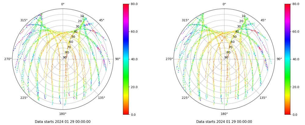
Skyplot for station LPAL. Parameter M1C Data file LPAL00ESP_R_2024029.xtr Skyplot for station LPAL. Parameter M2C Data file LPAL00ESP_R_2024029.xtr
