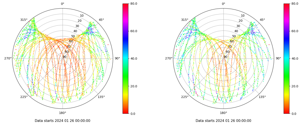
Skyplot for station LPAL. Parameter M1C Data file LPAL00ESP_R_2024026.xtr Skyplot for station LPAL. Parameter M2S Data file LPAL00ESP_R_2024026.xtr
