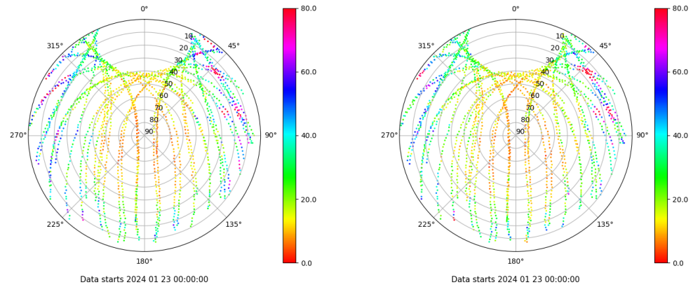
Skyplot for station LPAL. Parameter M1C Data file LPAL00ESP_R_2024023.xtr Skyplot for station LPAL. Parameter M2C Data file LPAL00ESP_R_2024023.xtr
