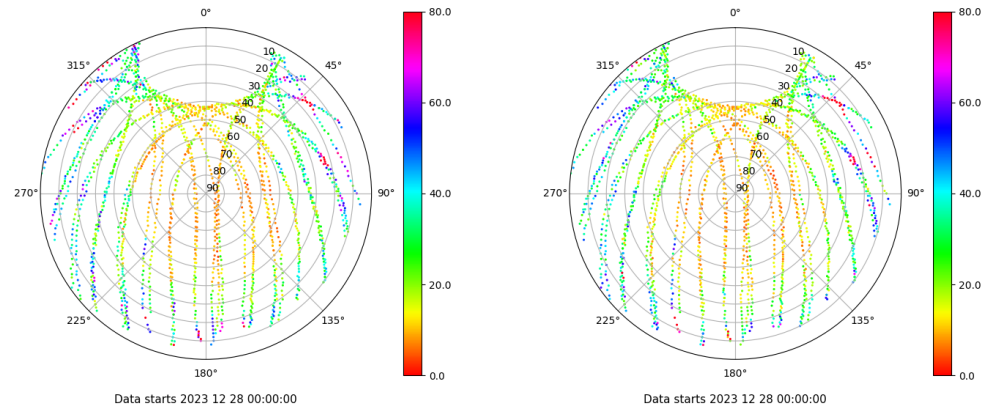
Skyplot for station LPAL. Parameter M1C Data file LPAL00ESP_R_2023362.xtr Skyplot for station LPAL. Parameter M2C Data file LPAL00ESP_R_2023362.xtr
