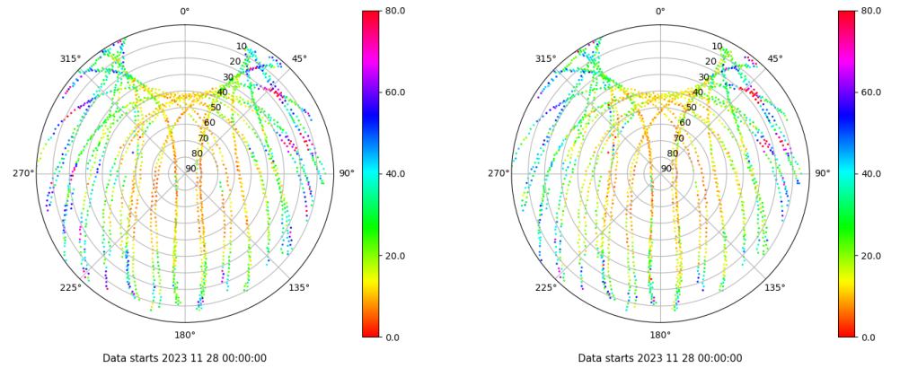
Skyplot for station LPAL. Parameter M1C Data file LPAL00ESP_R_2023332.xtr Skyplot for station LPAL. Parameter M2C Data file LPAL00ESP_R_2023332.xtr
