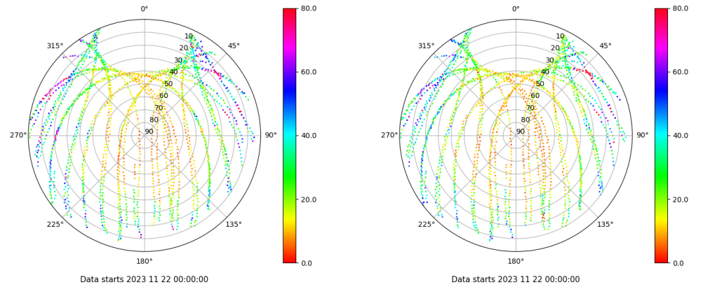
Skyplot for station LPAL. Parameter M1C Data file LPAL00ESP_R_2023326.xtr Skyplot for station LPAL. Parameter M2C Data file LPAL00ESP_R_2023326.xtr
