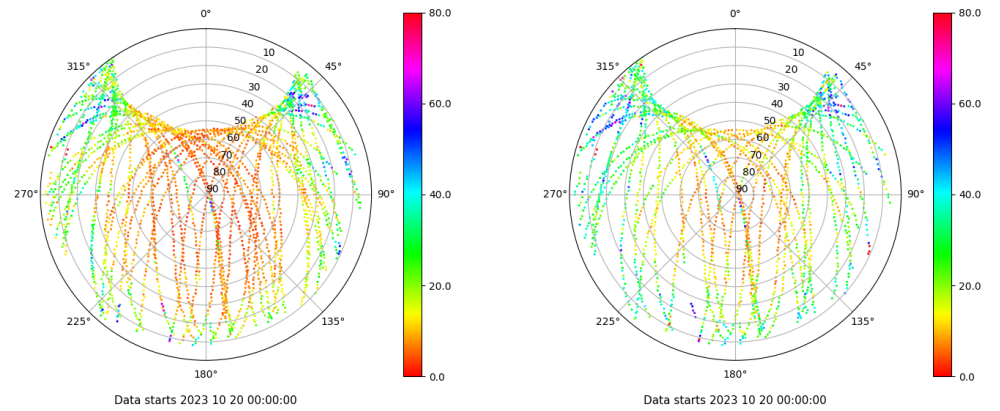
Skyplot for station LPAL. Parameter M1C Data file LPAL00ESP_R_2023293.xtr Skyplot for station LPAL. Parameter M2S Data file LPAL00ESP_R_2023293.xtr
