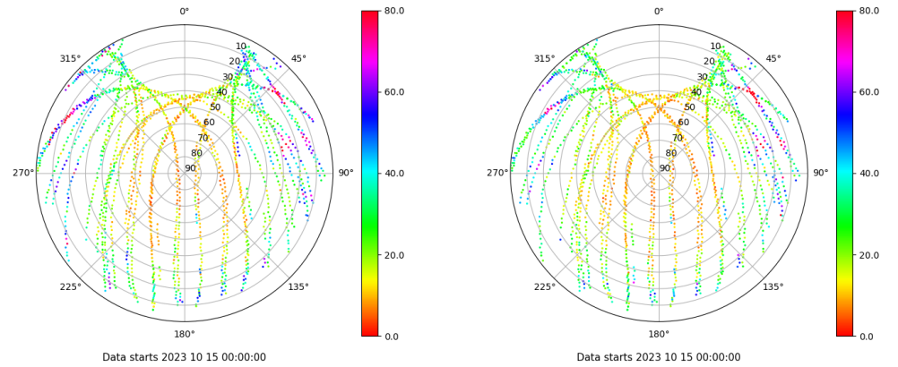
Skyplot for station LPAL. Parameter M1C Data file LPAL00ESP_R_2023288.xtr Skyplot for station LPAL. Parameter M2C Data file LPAL00ESP_R_2023288.xtr
