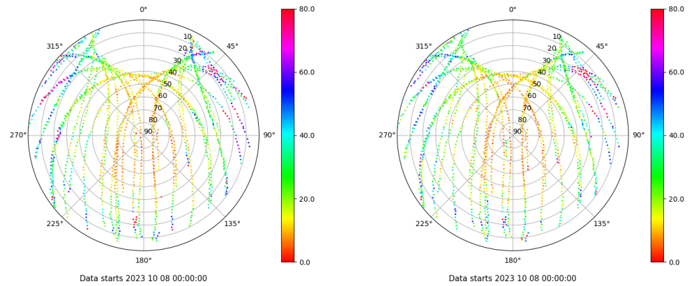
Skyplot for station LPAL. Parameter M1C Data file LPAL00ESP_R_2023281.xtr Skyplot for station LPAL. Parameter M2C Data file LPAL00ESP_R_2023281.xtr
