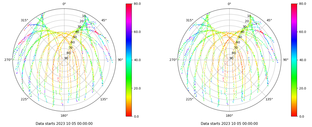
Skyplot for station LPAL. Parameter M1C Data file LPAL00ESP_R_2023278.xtr Skyplot for station LPAL. Parameter M2C Data file LPAL00ESP_R_2023278.xtr
